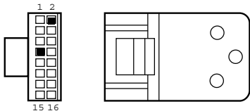
Figura 1. Bloque de conexión de 16 pines
