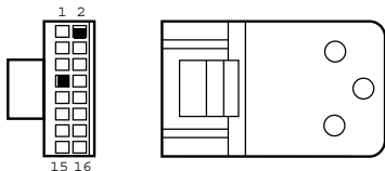
Afbeelding 1. 16-polige blokstekker
