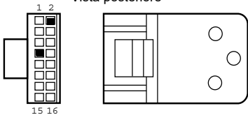
Figura 1. Basetta connessioni a 16 pin
