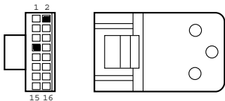
Рис. 1. 16-штырьковый разъем
